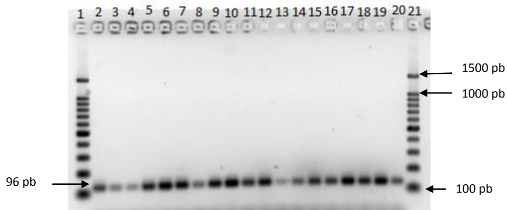
Figure 4: Produits d'amplification obtenus à partir des 18 colonies sélectionnées d' E.coli EC04 après 1 traitement (puits 3 à 11) et 8 traitements (puits 12 à 20) au Galox Horizon. Souche de référence E.coli ATCC25922 (puit 2). Marqueur de taille de 100 paires de bases (pb) (Promega) (puits 1 et 21).
