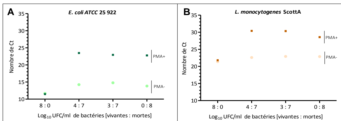
Figure 5 : Résultats des essais préliminaires de PCRq-PMA. Les essais diffèrent selon le ratio de bactéries vivantes et mortes, exprimé en log 10 UFC/ml de bactéries [vivantes : mortes] mais aussi selon l'ajout (PMA+ ; couleur foncée) ou non (PMA - ; couleur claire) de 50 µM de PMA.
