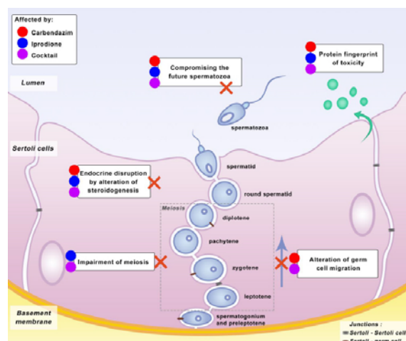
Illustration 38 : Coupe d'un tube séminifère indiquant les différents stades de la spermatogénèse et l'impact toxique des différents fongicides (Source : Odette Prat)
