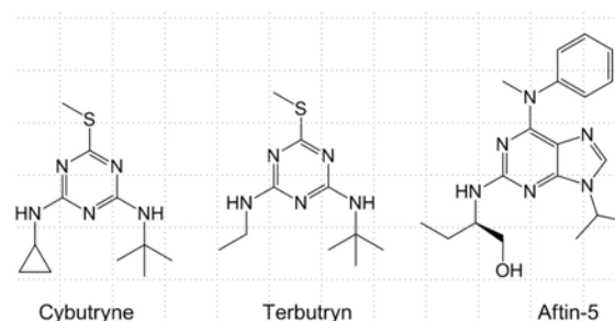
Illustration 57 : Structure des triazines inductrices de production d'amyloïdes Aβ-42. L'Aftine-5 est utilisée comme témoin positif 204
