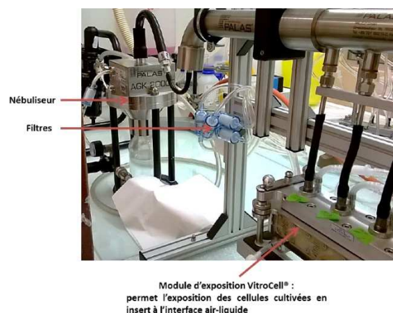
Illustration 25 : Modèle d'exposition à l'interface air-liquide (Source : BMBI/Ineris)
